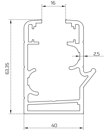
Damlalıklı Kasa Profili / Dropper Case Profile
