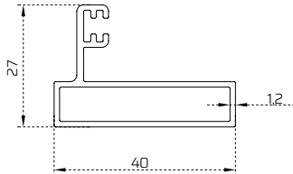
Yan Dikme Profili / Side Case Profile
